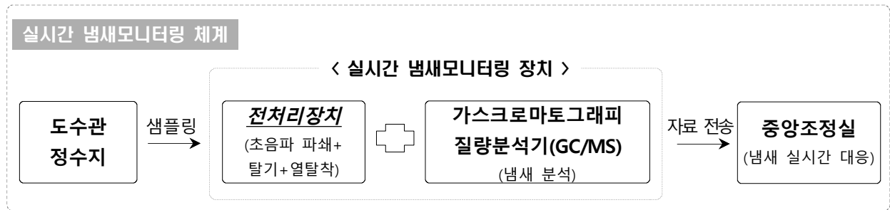
[그림 1] ∞ ∞ ∞ 지사 실시간 냄새물질 감시장치 모니터링 체계
